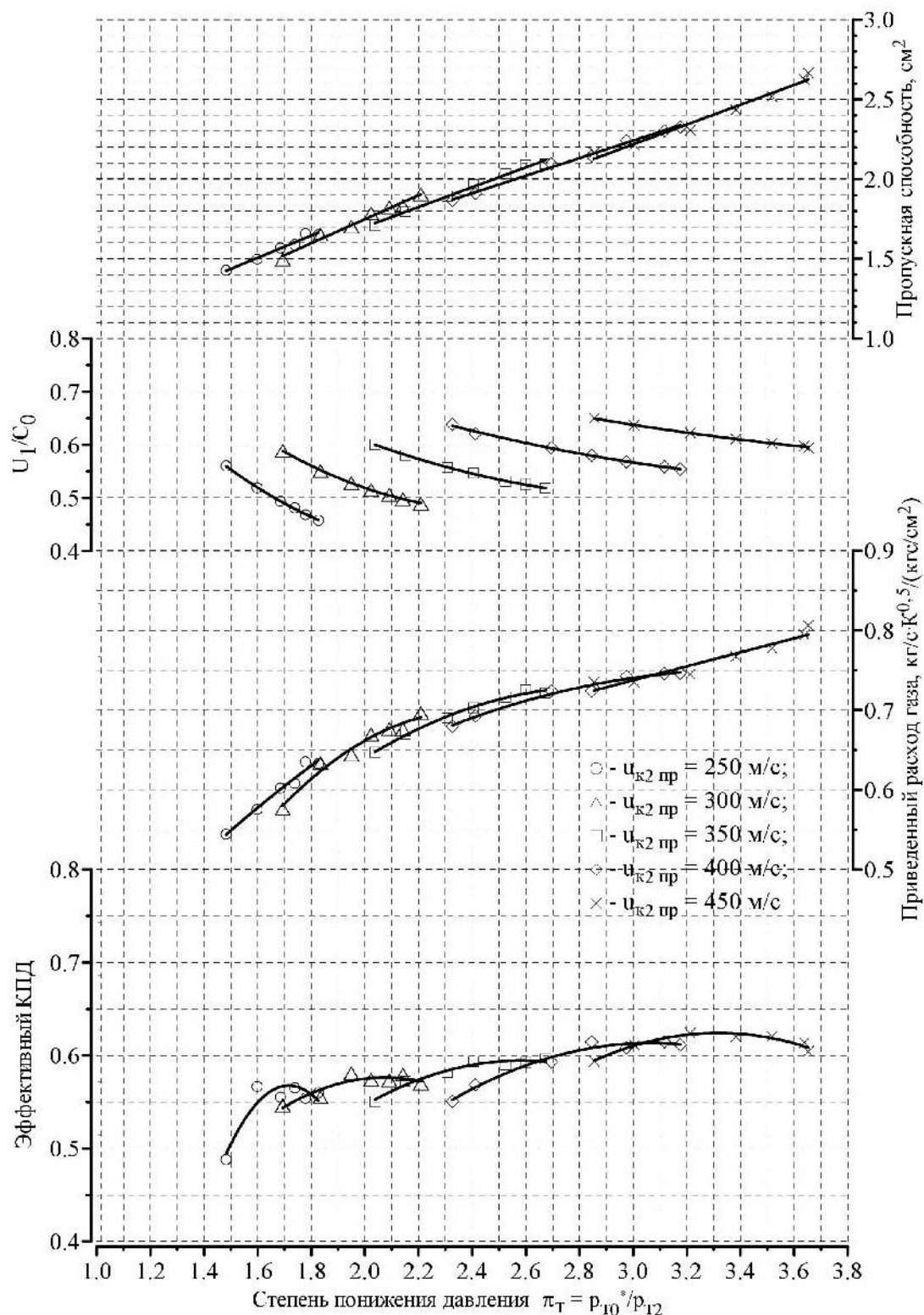
Характеристики турбины ТКР 50.01.03
